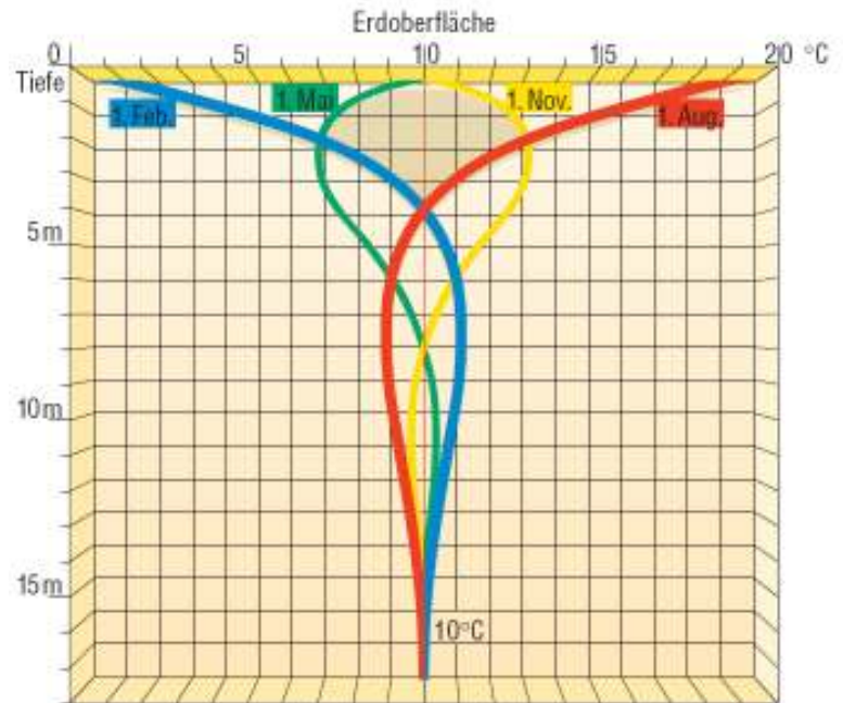
Mittlerer Temperaturverlauf im ungestörten Erdreich in Abhängigkeit von der Jahreszeit (Quelle: Bundesverband Wärmepumpe – BWP)
